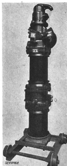
Fig. 5 Ölstrahlschalter HP 7 - 16% Hz für Innenraumaufstellung (Nennspannung 20 kV, Nennstrom 1000 A, Nennabschaltleistung 250 MVA bei 16 kV) Eingebaut als Fahrleitungs-Speisepunktschalter im Netz der SBB
