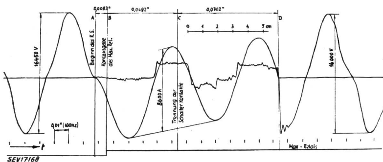
Fig. 4 Oszillogramm der Abschaltung eines Kurzschlussstromes von 8600 A bei 16 kV durch den Ölstrahlschalter HPF 7 - 16% Hz (Nennspannung 30 kV, Nennstrom 1000 A, Nennabschaltleistung 250 MVA bei 16 kV) Aufgenommen anlässlich der Abschaltversuche im Unterwerk Seebach der SBB A Beginn des Kurzschlussstromes; B Kontaktgabe des Maximal-Relais; C Trennung der Schaltkontakte; D Löschpunkt des Lichtbogens
