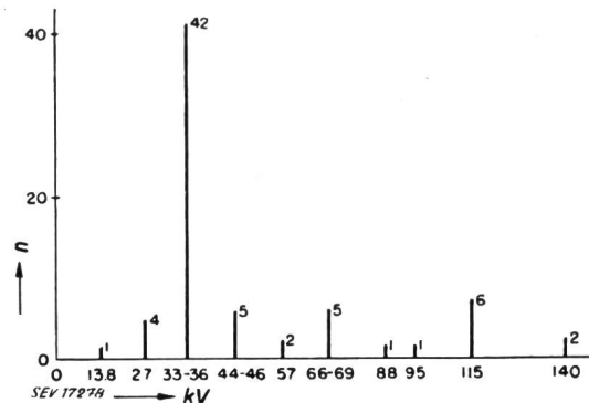
Fig. 3 Verteilung der 1946 in Amerika insgesamt betriebenen 69 Löschspulen auf die verschiedenen Spannungen n Anzahl der Löschspulen
