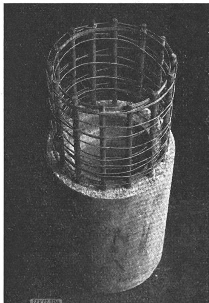
Fig. 2 Querschnitt durch Mast aus Schleuderbeton
