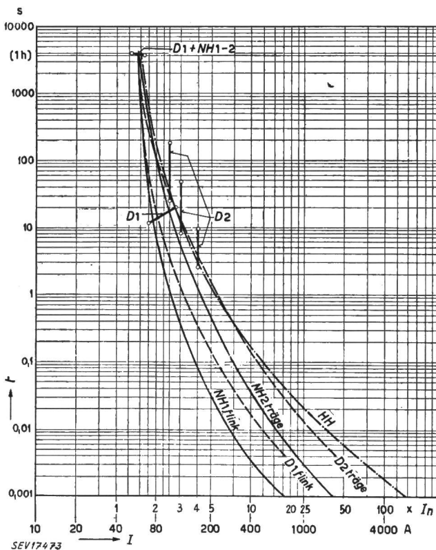
Fig. 3 Vergleich von Abschmelzcharakteristiken verschiedener Sicherungssysteme für einen 40-A-Schmelzleiter I Überstrom; I_n Nennstrom; t Abschmelzzeit; D1, Vorschrift des SEV für D1-Sicherungen; D2, Vorschrift des SEV für D2-Sicherungen; D1 + NH 1-2, Vorschrift des SEV für D1- und NH-1-2-Sicherungen
