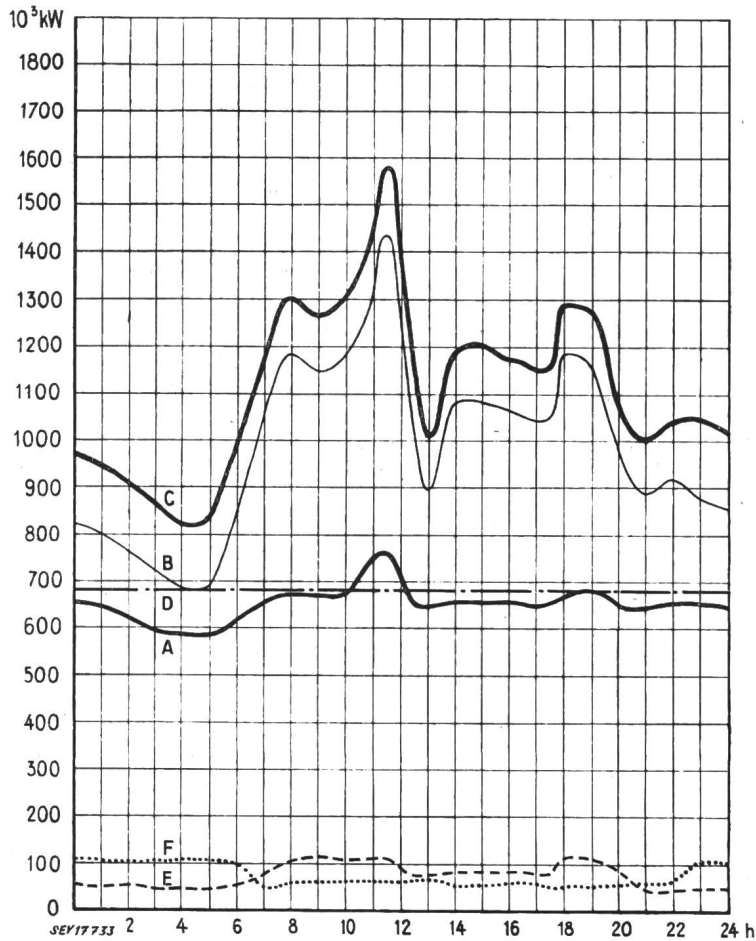
Diagramme de charge journalier du mercredi 18 octobre 1950
