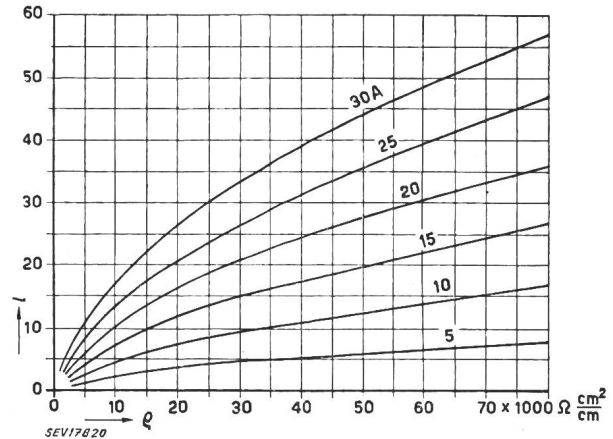
Fig. 20 Bandlänge in Abhängigkeit vom spezifischen Erdwiderstand für die Einhaltung der maximal zulässigen Belastung der Elektroden l Bandlänge; ρ spezifischer Erdwiderstand
