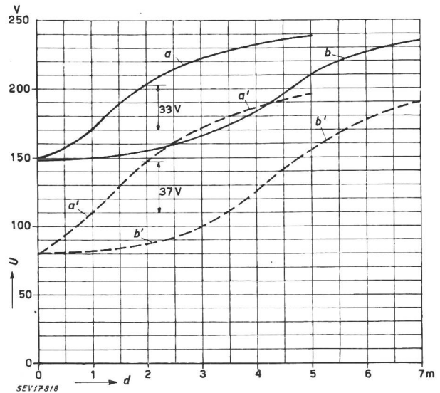
Fig. 18 Spannungsverlauf an der Erdoberfläche bei unveränderter Erdschlußstromstärke
