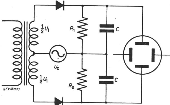
Fig. 11 Demodulator
