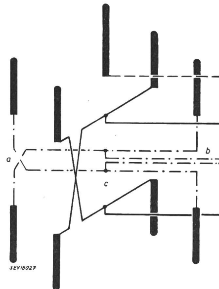
Fig. 5 Anordnung der Antennen eines Adcocksystems (räumliche schematische Darstellung, von der Seite gesehen) Je zwei gegenüberliegende Dipole sind durch eine Parallel- drahtleitung verbunden. In deren Mitte zweigt die Leitung zum Modulator ab. Im Zentrum der Dipolanordnung befindet sich die Referenzantenne
