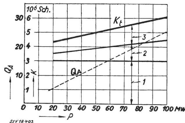
Fig. 3 Kosten eines Wasserkraftwerkes mit Jahresspeicherung und reiner Winterproduktion Q_A Ausbaumassmenge; K Jahreskosten in Millionen Schilling; K_t totale Jahreskosten; P installierte Leistung; Aufteilung der Jahreskosten: 1 Speicher, 2 Stollen, 3 Rohrleitung und Maschinenhaus
