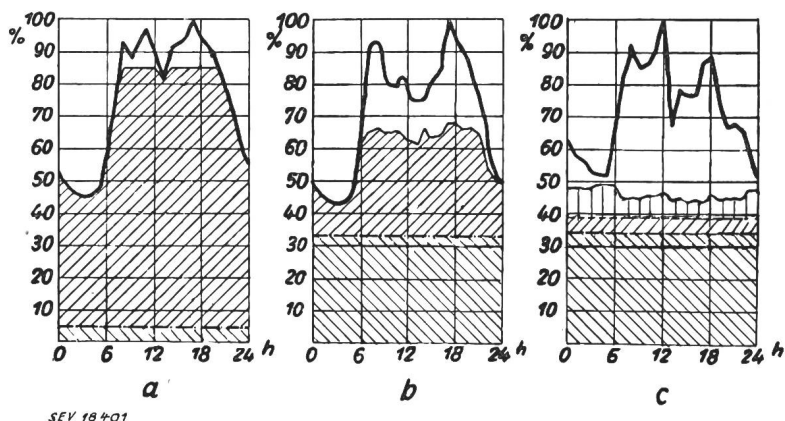
Fig. 1 Lastverteilungsdiagramme eines Wintertages a West-Deutschland, Dezembertag 1960; b Österreich, 15. Dezember 1949; c Schweiz, 14. Dezember 1949
