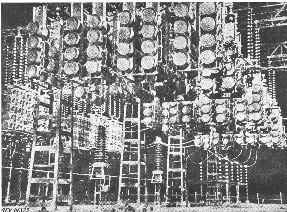
Teilansicht des Seriiekondensators in Alfta, Schweden
