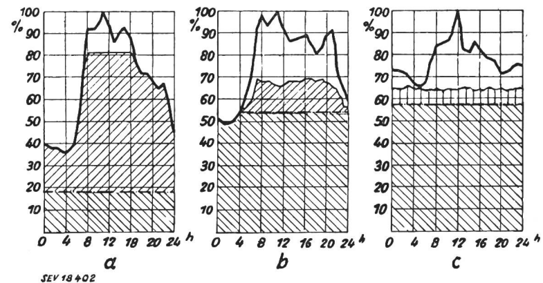
Fig. 2 Lastverteilungsdiagramme eines Sommertages a West-Deutschland, Julitag 1960; b Österreich, 16. Juli 1949; c Schweiz, 19. Juni 1949. Weitere Bezeichnungen siehe Fig. 1
