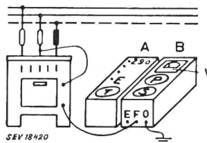
Fig. 9 Fehlerspannungsmessung bei direktem Erdschluss
