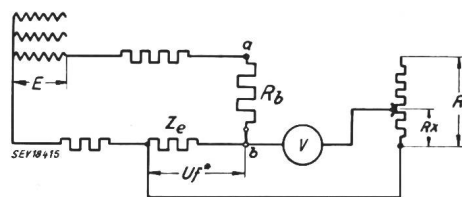
Fig. 4 Prinzipschema mit in der Fehlerstrombahn angeschlossenem EP-Gerät in Schalterstellung 3
