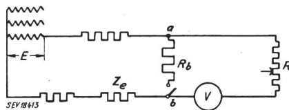
Fig. 2 Prinzipschema mit in der Fehlerstrombahn angeschlossenem EP-Gerät in Schalterstellung 1
