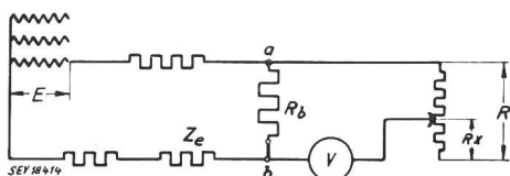
Fig. 3 Prinzipschema mit in der Fehlerstrombahn angeschlossenem EP-Gerät in Schalterstellung 2
