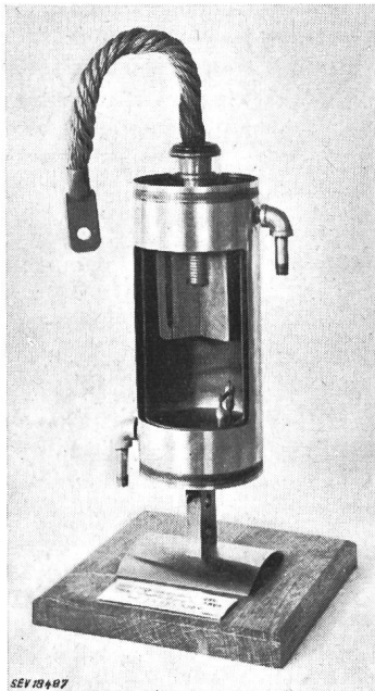
Fig. 1 Ignitron Schalteröhre Maximale Schaltleistung 1200 kVA
