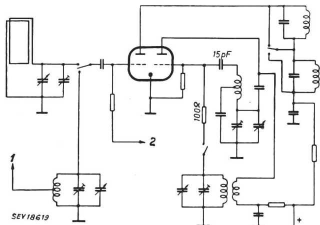
Fig. 6 Amerikanische Mischstufe für UKW- und Mittelwellenempfang mit Doppeltriode als Mischrohr 1 zur FM-Antenne; 2 zum Regelkreis
