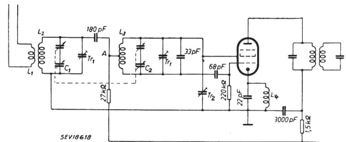
Fig. 5 Additive Mischung und Schwingungserzeugung in einer Röhre
