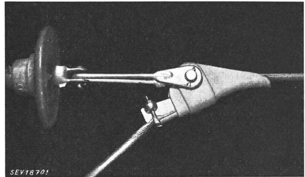
Fig. 3 Leichte Abspannklemme Konstruktion AIAG
