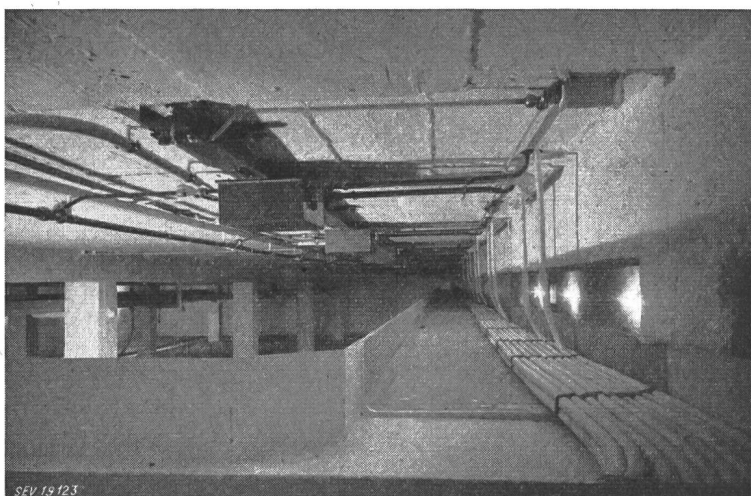
Fig. 6 Anordnungen der Druckluftleitungen und Steuerkabel unter der 16-kV-Schaltanlage
