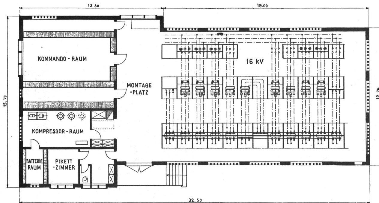
Fig. 4 Grundriss des 16-kV-Schalthauses
