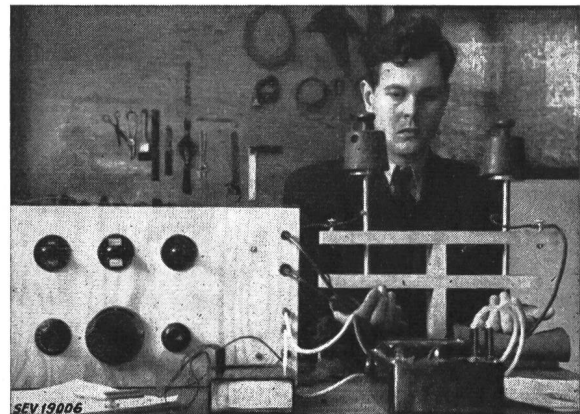
Fig. 6 Messanordnung
