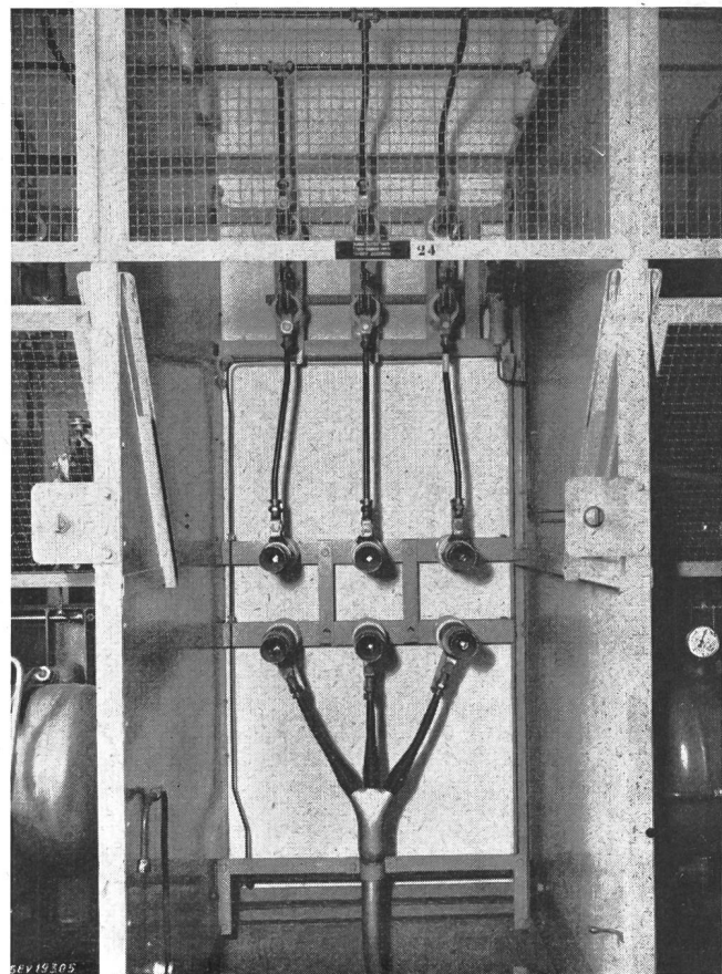
Fig. 5 Einbauzelle mit festen Tulpenkontakten
