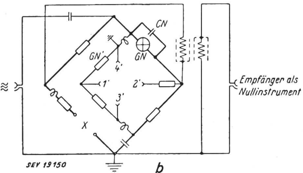
Fig. 5 Brückenmessung von Scheinwiderständen mit gesteuertem Widerstandsnormal a) Brücke für kleine Leitwerte b) Brücke für kleine Widerstände Erläuterungen siehe im Text
