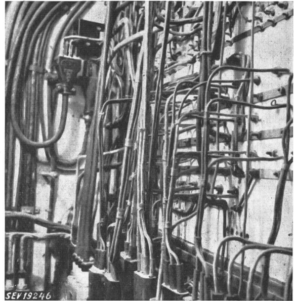
Fig. 35 Ancienne installation de distribution d'une entreprise industrielle
