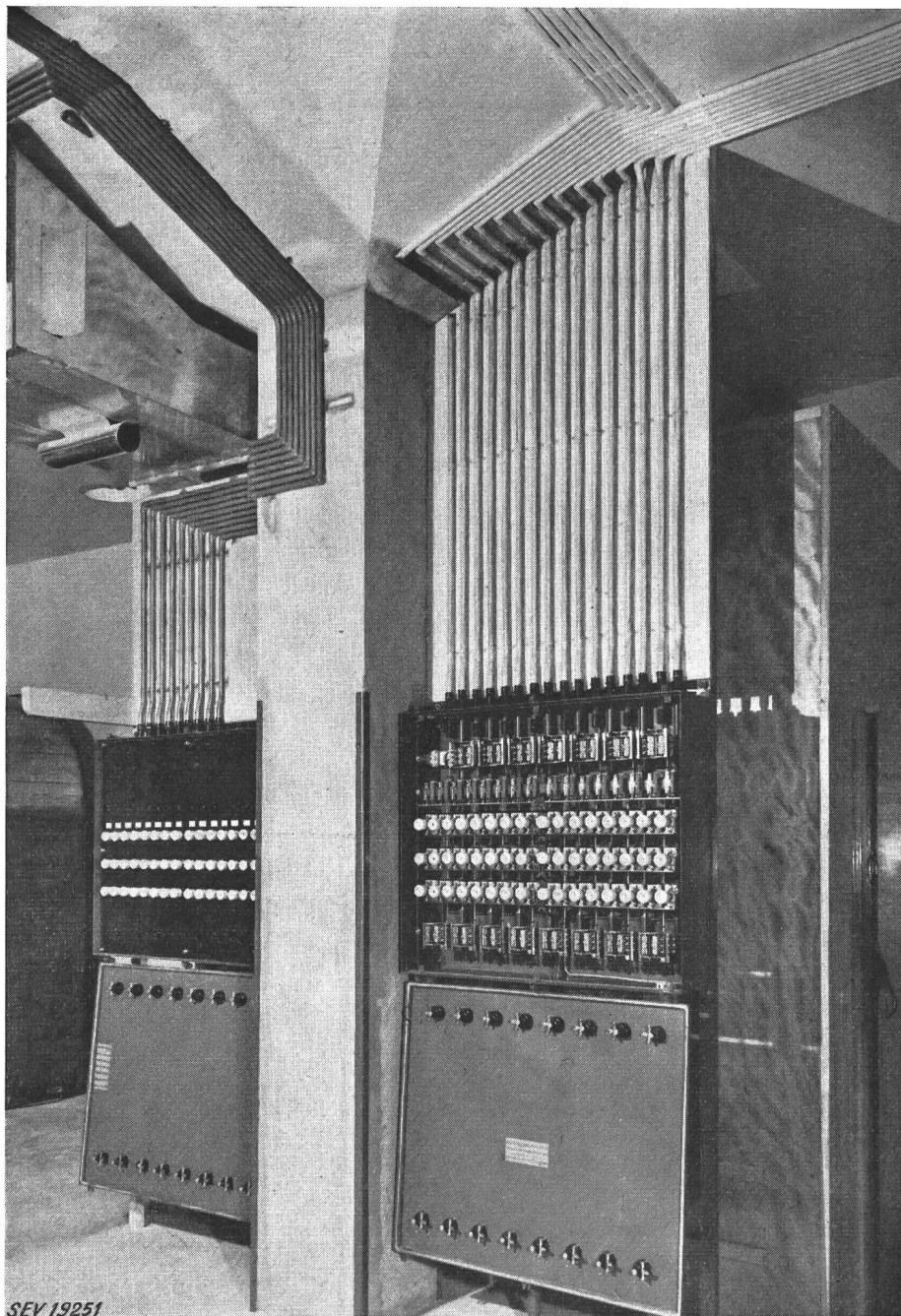
Fig. 40 Appareillage de distribution blindé Installé en 1951
