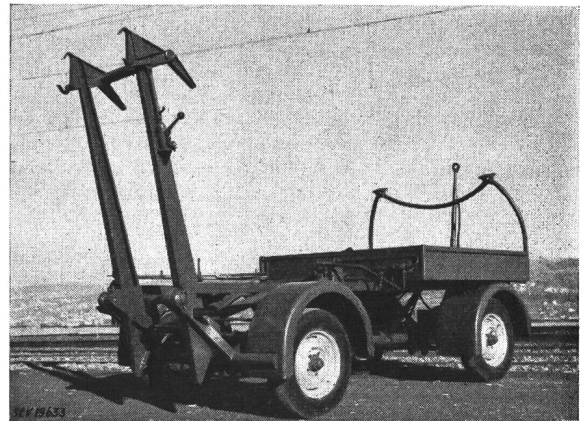
Fig. 5 Anhänger für Strassentransport von Rolleitern
