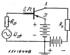
Fig. 5 Steuer-spitzen-Basis-schaltung eines Transistors
