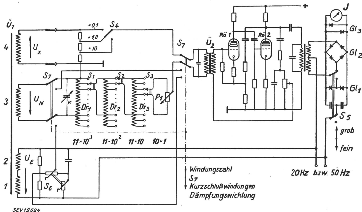
Fig. 2 Prinzipschema für Windungszahl- und Kurzschlusswindungsmessung
