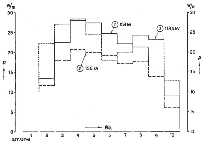
Fig. 10 Répartition longitudinale des pertes par effet de couronne. Tube de cuivre de 25 mm \phi . 1 à sec, le matin du 7. 11. 51, sous 158 kV; 2 à sec, le soir, du 7. 11. 51, sous 156 kV; 3 sous pluie irrégulièrement répartie, le 16. 11. 51, sous 118,5 kV
