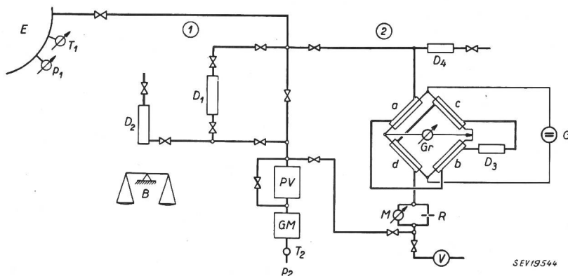
Fig. 11 Mesure de l'humidité ① Méthode de mesure par absorption; ② Méthode de mesure au pont (BBC); E Enceinte climatique étanche; PV Pompe à haut vide; GM Gazomètre; D1...D4 Dessiccateurs; p1, p2, M Manomètres; T1, T2 Thermomètres; G Source de courant; Gr Instrument de mesure (g/m 3 ); a, b, c, d Branches du pont; R Diaphragme; V Ventilateur; B Balance de précision (Sensibilité 2 mg, tare 500 g)
