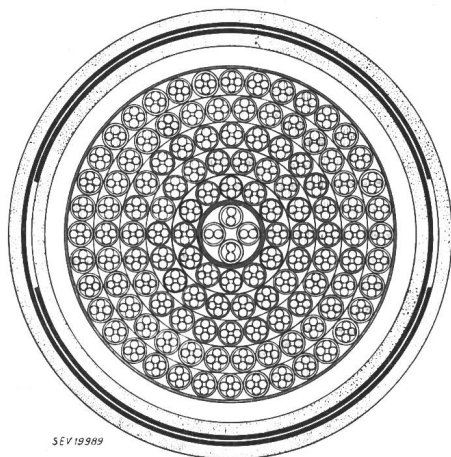
Fig. 4 Bezirks- oder Fernkabel in Sternviererverseilung mit 244 \times 2 Adern von 1,0 mm \phi (120 Vierer und 4 Musikpaare)
