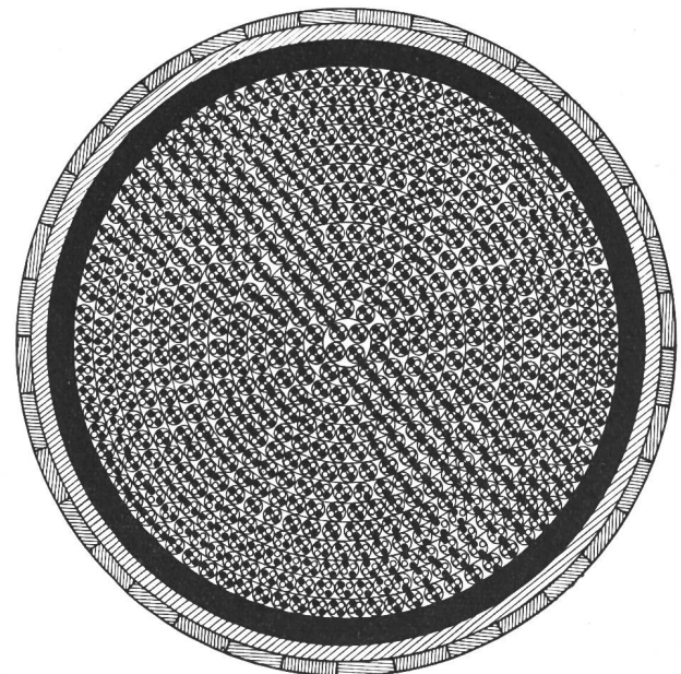
Fig. 5 Teilnehmer- oder Abonnenkabel in Sternviererverseilung mit 1204 \times 2 Adern von 0,6 mm \phi (600 Vierer und 2 Reservevierer)
