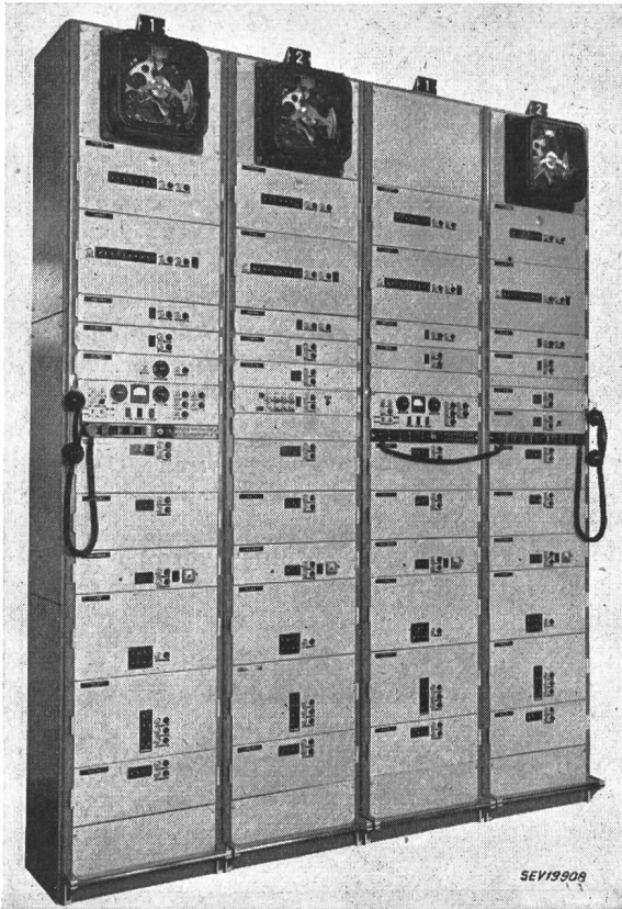
Fig. 7 Zwischenstation einer Richtstrahl-Verbindung für die Saudi-Arabian Railroad
