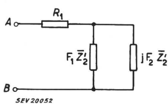
Fig. 10 Schéma équivalent d'une impédance négative-parallèle R_1 résistance compensatrice de \bar{Z}_a (cf. fig. 6 et 7) F_1 et F_2 fonctions caractéristiques de l'amplificateur, définies par équation (38) Z'_2 = \bar{Z}_2 + \bar{Z}_a (cf. fig. 6 et 7)
