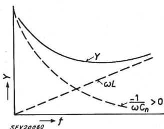
Fig. 18 Positance-série Connection-série d'une inductivité positive L et d'une capacité négative C_n
