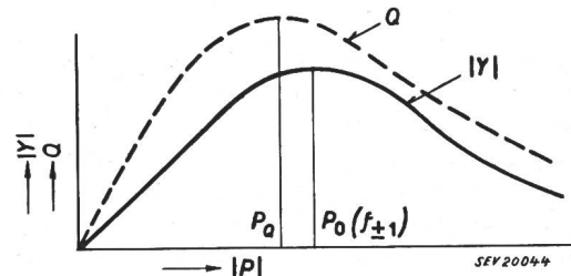
Fig. 2 Représentation graphique de la valeur absolue |Y| de la réactance négative Y d'un tube-réactance, et de son coefficient de qualité Q en fonction de la valeur absolue |P| de la réactance transformée P
