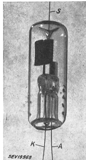
Fig. 7 Glimmrelais des Feuermelders Bezeichnungen siehe im Text
