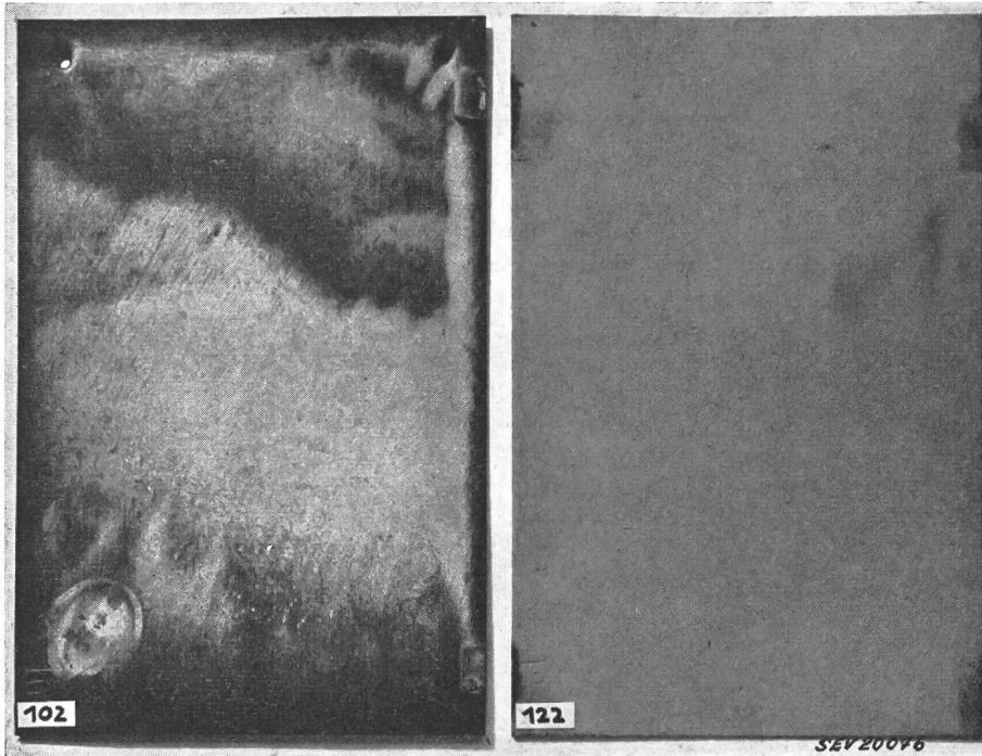
Fig. 1 Bleche der Versuchsstation Dietikon (7 Jahre Pendelwässerung) a Nr. 102 (vollbadverzinkt), vereinzelte Rostpunkte b Nr. 122 (spritzverzinkt), keine Rostbildungen
