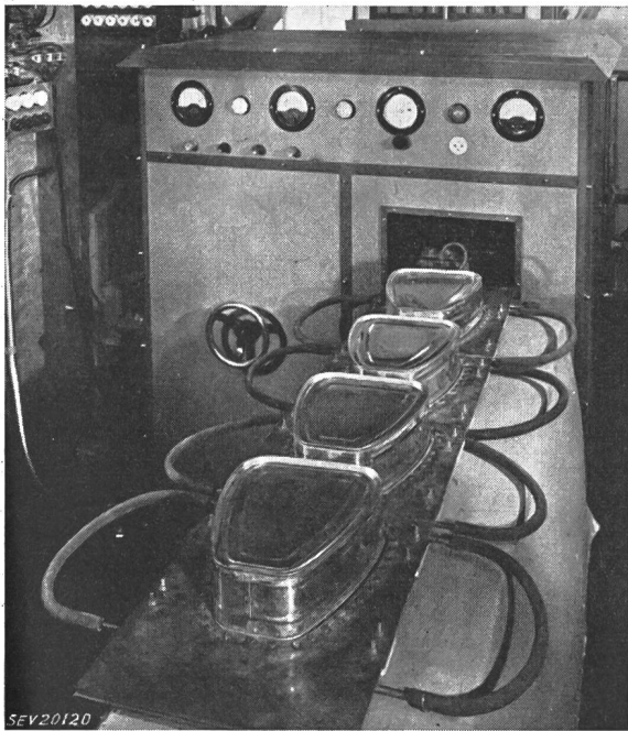
Fig. 10 Verlöten von Konservbüchsen Vier von den in Fig. 9 abgebildeten Kupferplatten werden in Serie als Arbeitsspule verwendet
