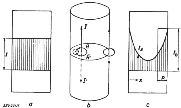
Fig. 1 Skineffekt (Stromverdrängung)
