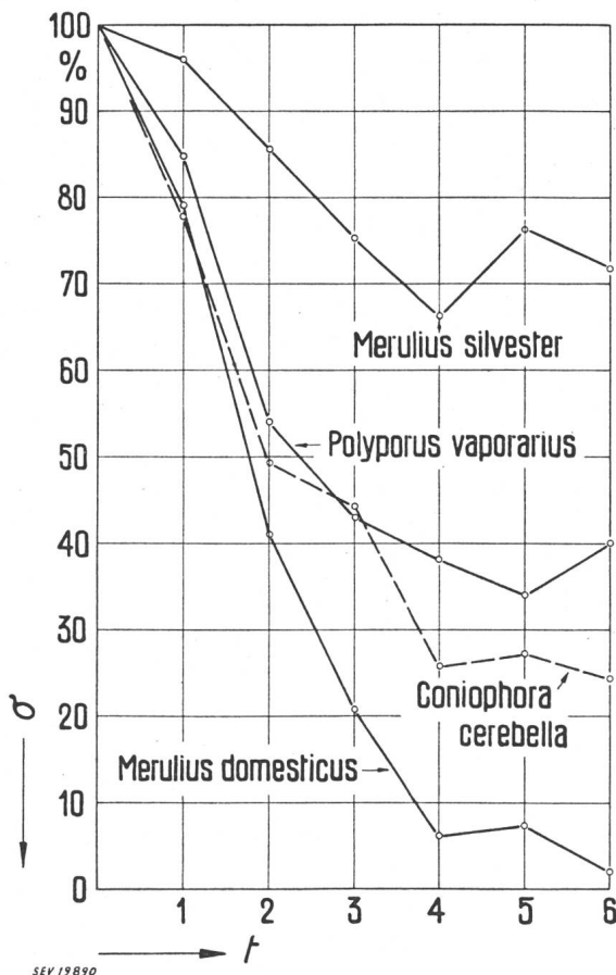
Fig. 8 Diminution de la résistance du bois de pin causée par l'action plus ou moins longue de champignons lignivores \sigma résistance restante; t temps d'action en mois
