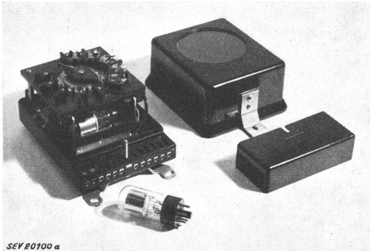
Netzkommandoempfänger mit Glimmrelais Dem Netz überlagerte Tonfrequenz (ca. 1...2 kHz, 1...2 V) fließt durch den Kondensator C und die Primärwicklung des Resonanztransformators T. Sekundärseitig wird die Tonfrequenzspannung auf etwa 150 V transformiert. Sie zündet die Steuerstrecke KS und diese die Hauptstrecke KA des Glimmrelais. Dessen Anodenstrom betätigt das Relais Re und dieses den Schaltmechanismus
