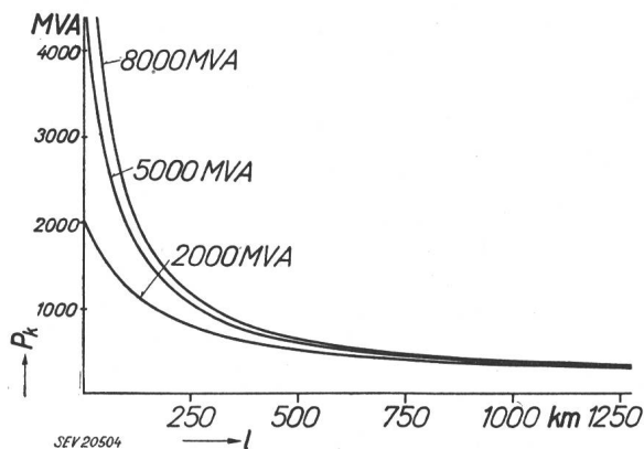
Fig. 1 Kurzschlussesleistungen längs einer 380-kV-Leitung P_k Abschaltleistung bei P_n \approx 400 MW natürlicher Leistung und Z = 375 \Omega Wellenwiderstand; l Leitungslänge
