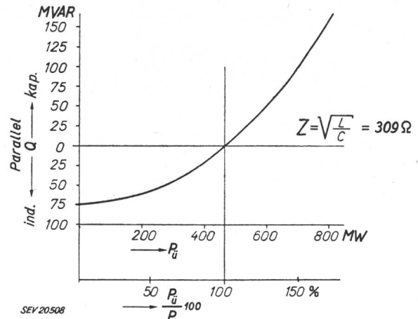
Fig. 5 Blindleistungsbedarf einer 380-kV-Leitung für gleiche Spannung am Anfang und Ende der Leitung Kompensationsmittel am Ende der Leitung angeschlossen Z Wellenwiderstand; Q Blindleistung; P_n übertragene Leistung am Leitungsende; P_n natürliche Leistung
