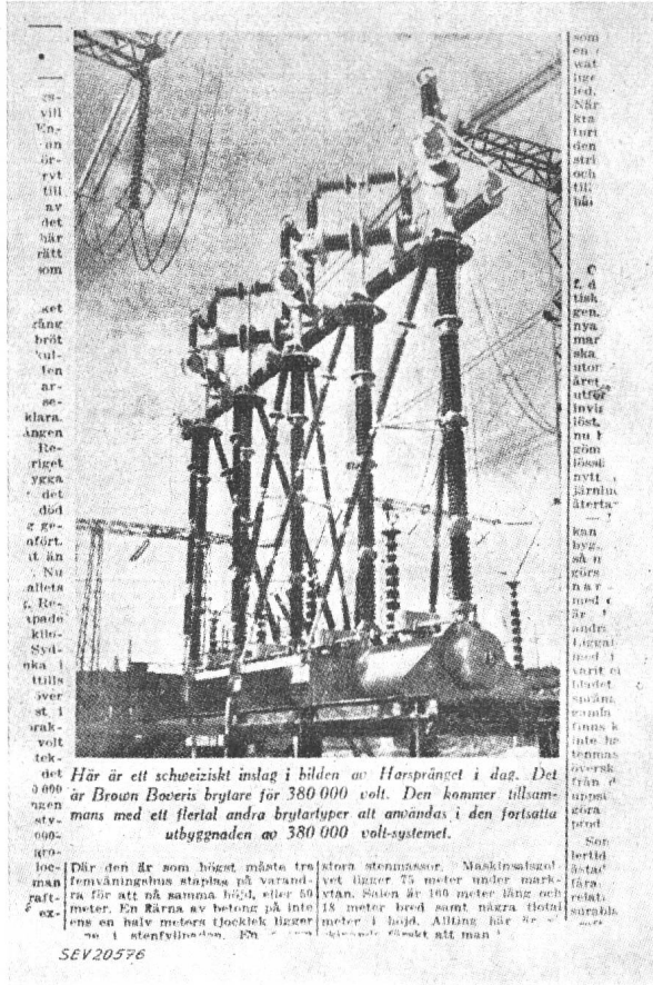
Fig. 9 Der 380-kV-Druckluftschalter Brown Boveri im Spiegel der schwedischen Presse (Sonderausgabe des «Svenska Dagbladet» vom 14. Juni 1952 zur offiziellen Eröffnung des Kraftwerkes Harsprånget durch den schwedischen König)
