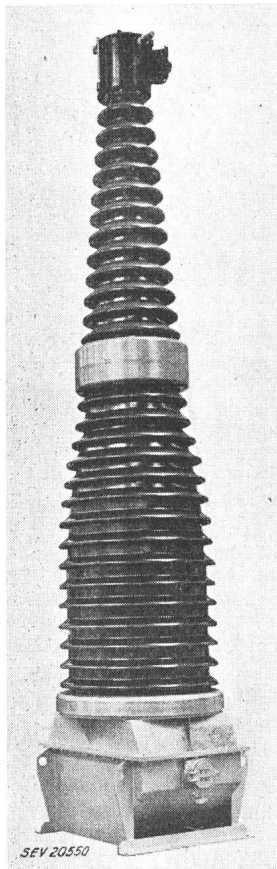
Fig. 1 Stromwandler 380 kV Nennspannung Bauart Maschinenfabrik Oerlikon, Zürich
