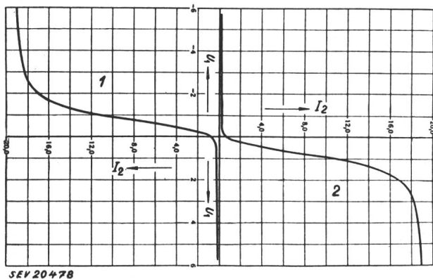
Fig. 2 Verstärkercharakteristik
