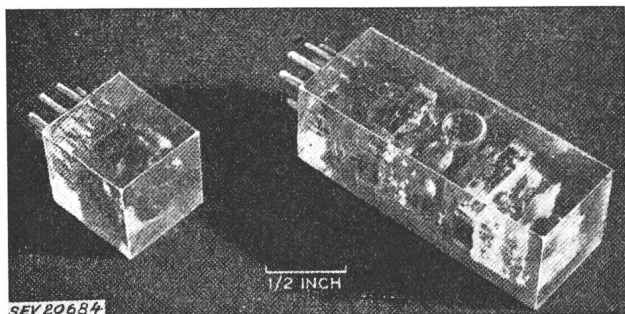
Fig. 5 Beispiel eines Verstärkers und eines Oszillators, bestückt mit Junction-Transistoren
