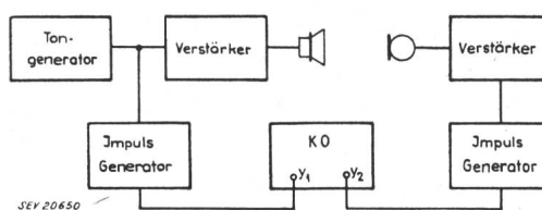
Fig. 1 Blockschema der Messeinrichtung
