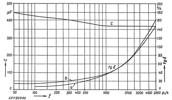
Fig. 7 Condensateur électrolytique STR Variation de la capacité C et de la \text{tg } \delta en fonction de la fréquence f a Condensateur régénéré (Mesure des ACO) b Condensateur neuf (Mesure de la Standard Telephon und Radio A.-G., Zürich)
