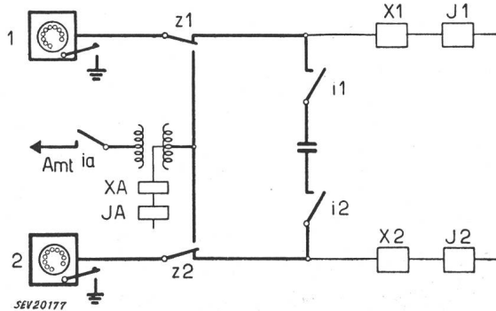
Fig. 2 Prinzipisches Schaltbild der Relaiszentrale I/2 Bezeichnungen siehe im Text
