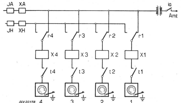
Fig. 3 Prinzipisches Schaltbild der Relaiszentrale I/6 Bezeichnungen siehe im Text
