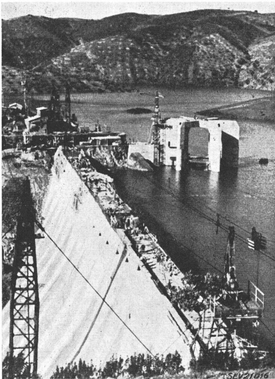
Fig. 4 Barrage à contreforts de Pracana (Portugal) et évacuateur de crue (crue de 150 m 3 /s avant l'achèvement des travaux) La vanne de l'évacuateur n'est pas encore montée. Capacité d'évacuation maximum: 1650 m 3 /s
