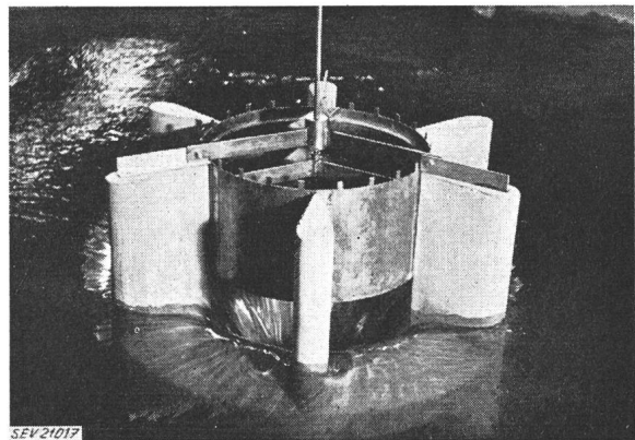
Fig. 5 Modèle de l'évacuateur du barrage de Pracana. Déversement d'un débit correspondant à 1000 m 3 /s
