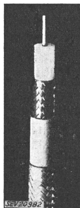
Fig. 9 Câble coaxial à isolation polythène muni d'une armure en fils d'acier (type RG 18 U)
