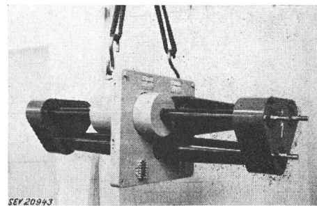
Fig. 13 Kombiniertes Spannungs-Stromwandler von 60 kV Spannungswandler-Wicklung in Kunstharz eingebettet
