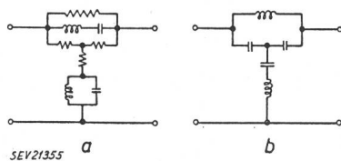
Fig. 15 Entzerrnetzwerke für Koaxialkabelleitungen a Dämpfungsentzerrer; b Laufzeitentzerrer
