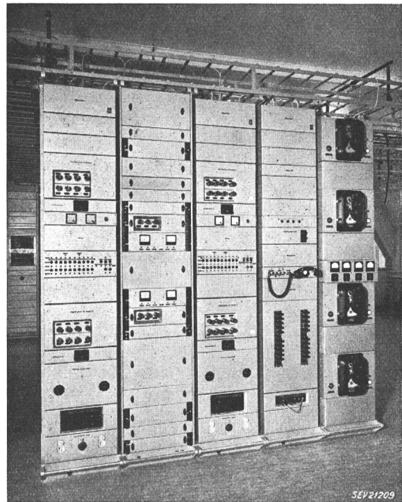
Fig. 8 Hauptamt Neuenburg, Linienrüstung
