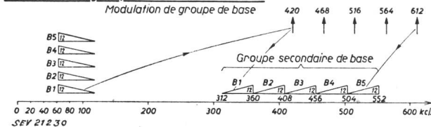
Fig. 2 Systèmes à modulation directe Formation d'un groupe secondaire de base
