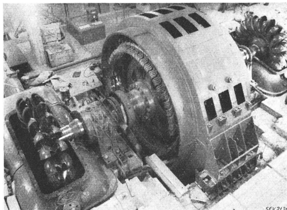
Fig. 1 Maschinenaal Grimsel des Kraftwerkes Oberaar Montagezustand am 13. Januar 1953
