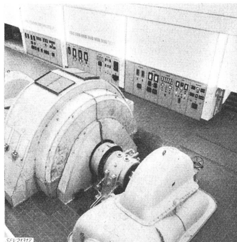
Fig. 2 Maschinenaal Grimsel des Kraftwerkes Oberaar Teilansicht des Maschinenaales bei der Betriebsaufnahme am 26. August 1953
