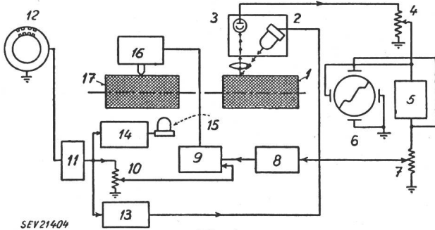
Fig. 4 Blockschema des elektronischen Graveurs 1 Abtastzylinder; 2 Abtastlichtquelle; 3 Photozelle; 4 Weiss-Kontrastkontrolle; 5 Gammakorrektur; 6 Kontroll-Kathodenstrahl-Oszillograph; 7 Gammakorrektur-Verstärkungskontrolle; 8, 11, 13, 14 Verstärker; 9 Kraftverstärker; 10 Schwarz-Kontrastkontrolle; 12 Rastergenerator; 15 Mikroskop-Lichtquelle; 16 Graveur mit Stichel; 17 Cliché-Zylinder
