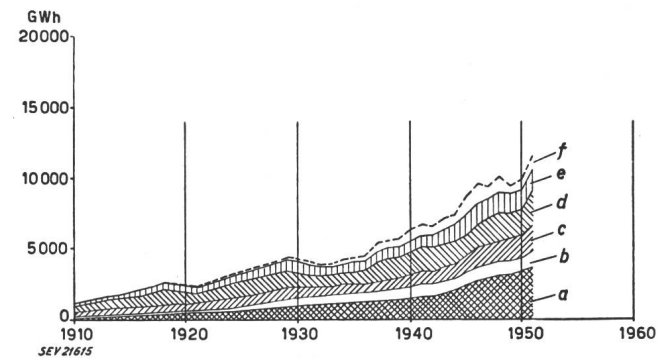
Fig. 5 Consommation suisse d'énergie brute en GWh électrique (prise à l'usine) a usages domestiques et artisanat; b traction; c industrie générale; d chimie et métallurgie; e pertes et énergie de pompage; f chaudières électriques
