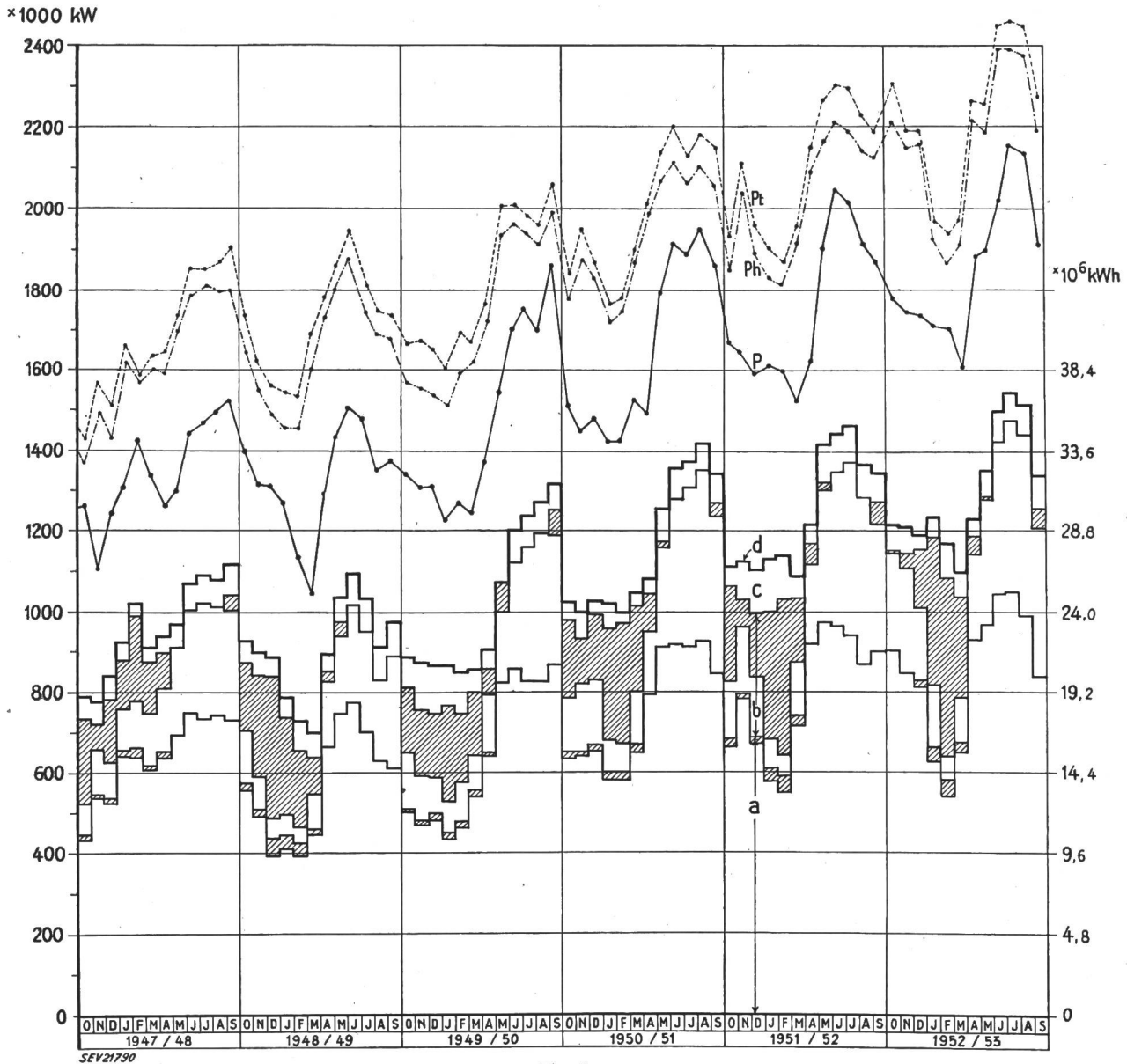
Fig. 8 Production mensuelle d'énergie et puissances maxima
