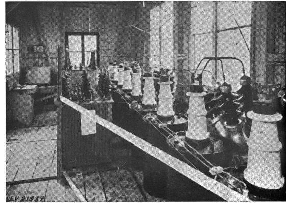
Fig. 5 Prüfeinrichtungen für die Dauerversuche
