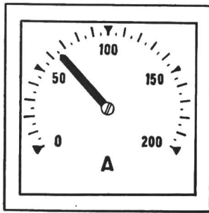
Fig. 5 Quadratisches Schalttafelinstrument mit zentraler Ringskala von 250°
