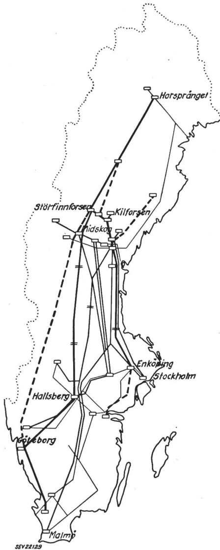
Fig. 1 Gegenwärtige Ausbreitung des 380-, 220- und 130-kV-Netzes mit den geplanten Ergänzungen
