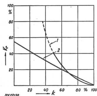
Fig. 2 Preiserhöhung bei herabgesetzter Reaktanz für Wasserkraftgeneratoren und Wert der Stabilität bei reduzierter Reaktanz K_r , relative Kostenänderung; k Übergangsreaktanz im Verhältnis zum normalen Wert; 1 Kosten der Synchronmaschine; 2 Wert der Stabilitätserhöhung
