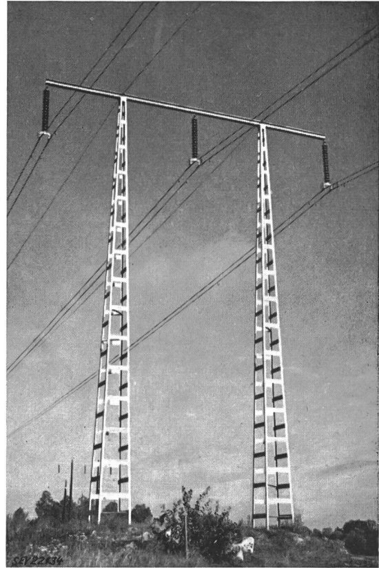
Fig. 6 220-kV-Leitung mit Bündelleitern
