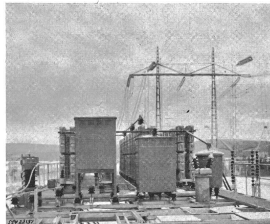
Fig. 9 Detail aus der 380-kV-Kondensatorstation
