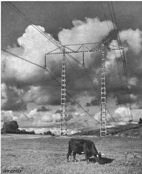
Fig. 5 380-kV-Leitung mit Bündelleitern
