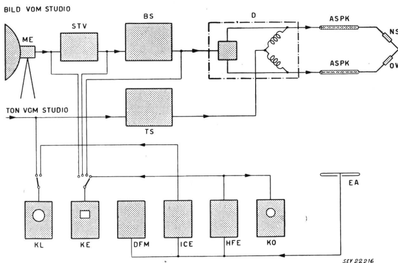
Fig. 4 Blockschma der Sendeanlage auf dem Uetliberg
