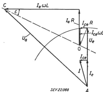
Vektordiagramm einer Fernleitung entsprechend dem Ersatzbild in Fig. 1 \text{tg } \epsilon = R/\omega L Weitere Bezeichnungen siehe Fig. 1 und Text
