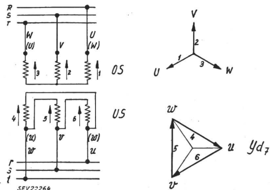
Fig. 5 Schaltgruppe eines Transformators mit der Wicklungsschaltung Yd5 (C2), bei vertauschten Anschlüssen R, S, T; r, s, t Pole des Drehstromsystems U, V, W Phasenbezeichnungen der Oberspannungen u, v, w Phasenbezeichnungen der Unterspannungen (U), (V), (W) Klemmen der Oberspannungswicklungen (u), (v), (w) Klemmen der Unterspannungswicklungen OS Oberspannungsseite US Unterspannungsseite 1...6 Bezugspfeile und Spannungsvektoren
