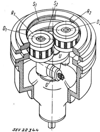
Ausführungsskizze eines Drehstrom-Rollstromrichters in Innenrollenauführung
