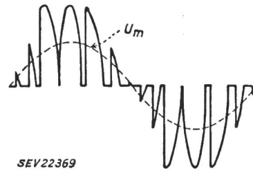
SEV 22369 Fig. 2 Ungesiebte Spannung an der Sekundärwicklung des Ausgangstransformators
