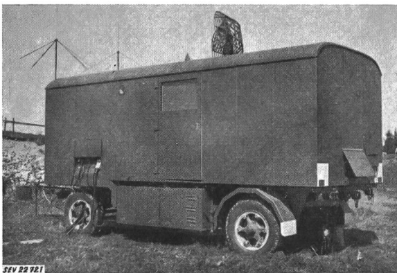
Fig. 21 Flab-Kommando-Zentrale (Schweiz)
