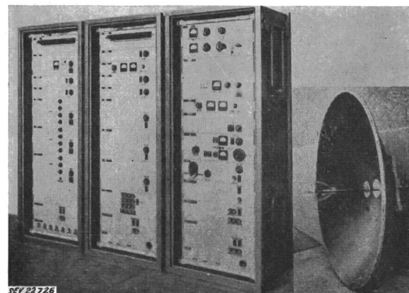
Fig. 26 Ultrakurzwellen-Richtstrahl-Mehrkanal-Funkgerät (Schweiz)
