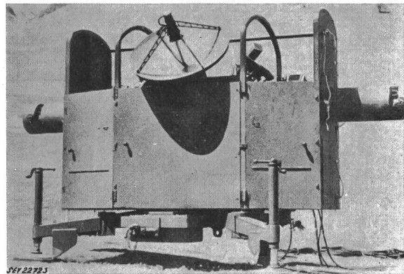
Fig. 23 Feuerleit-Radargerät Reichweite ca. 30 km (Schweiz/Frankreich)
