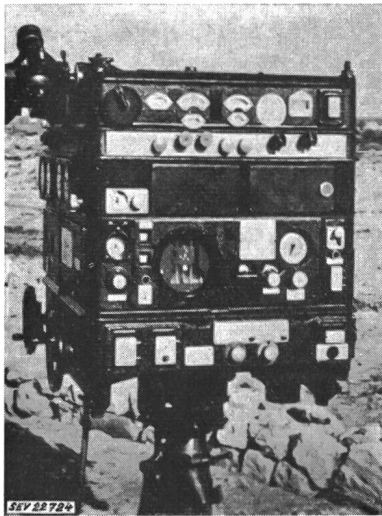
Fig. 24 Kommando-Gerät, mechanisch bei der Truppe eingeführt (Schweiz)
