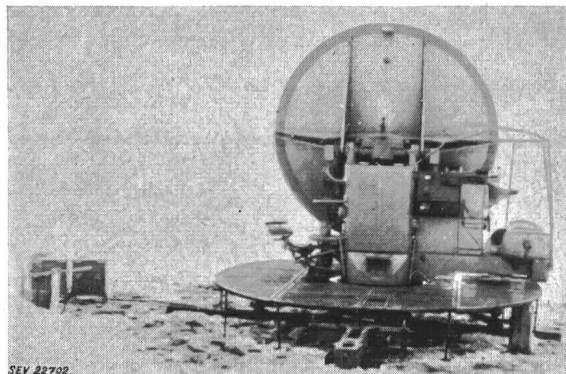
Fig. 2 Erprobung des deutschen Feuerleitradars «Würzburg-Dora» in der Schweiz im Jahre 1945
