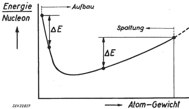
Fig. 2 Mittlere Bindungsenergie E der Kerne (pro Nucleon) als Funktion des Atomgewichtes A
